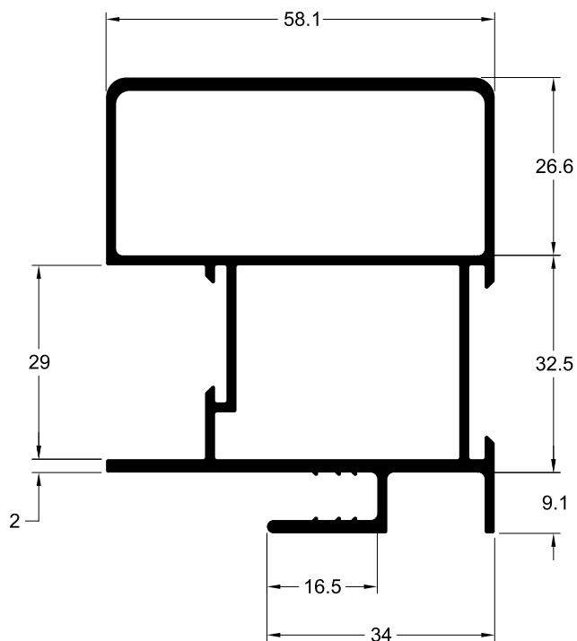
TLG-018 1.522 Kg/m
