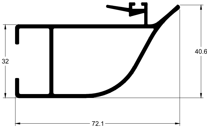
AG-035SB 0.931 Kg/m
