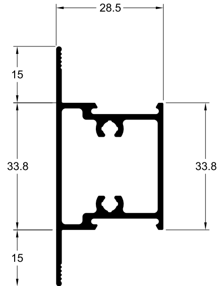
TLG-055 0.758 Kg/m
