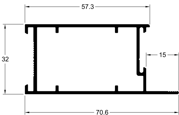
TLG-043R 0.807 Kg/m
