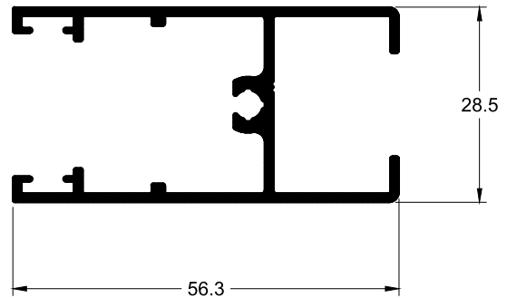
TLG-130 0.655 Kg/m
