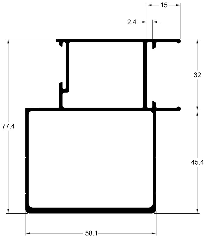
TLG-054 1.574 Kg/m
