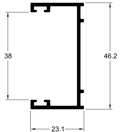
TLG-028 0.433 Kg/m
