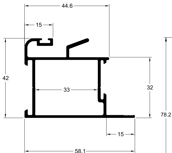
TLG-077C 0.890 Kg/m
