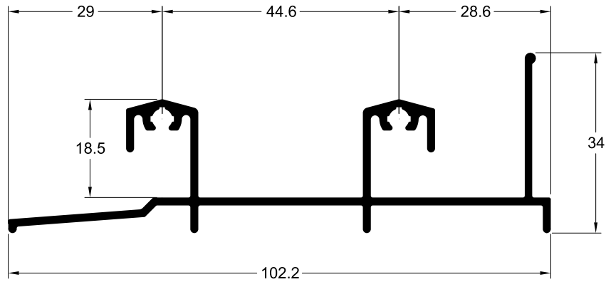
TLG-610 0.967 Kg/m
