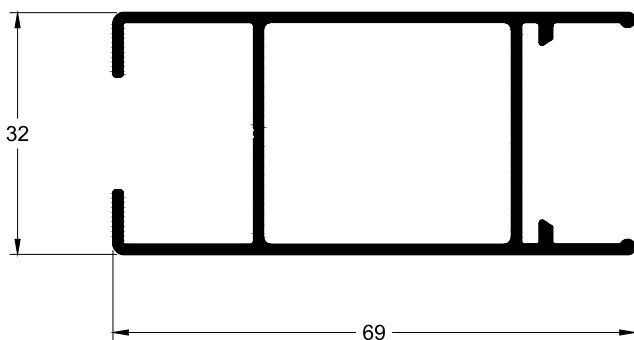
TLG-132 0.773 Kg/m
