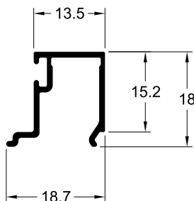
TBG-057 0.168 Kg/m
