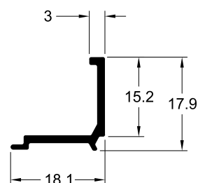
TLG-015 0.142 Kg/m
