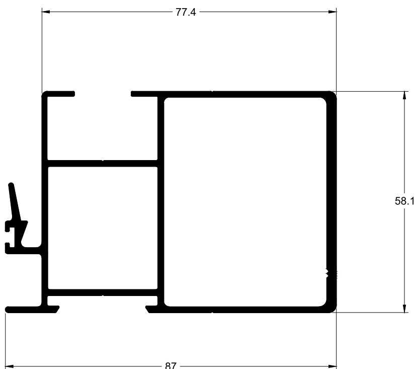
TLG-127A 1.698 Kg/m
