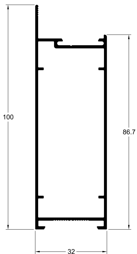
TLG-042 0.959 Kg/m
