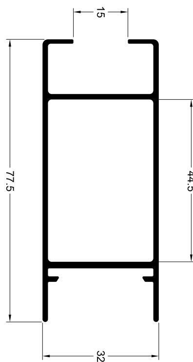
LG-34SB 0,957 Kg/m
