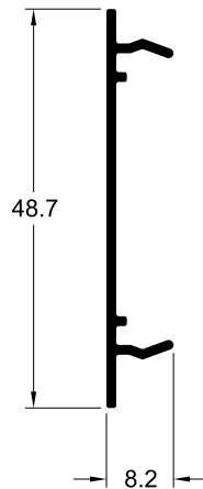
TLG-046 0.213 Kg/m
