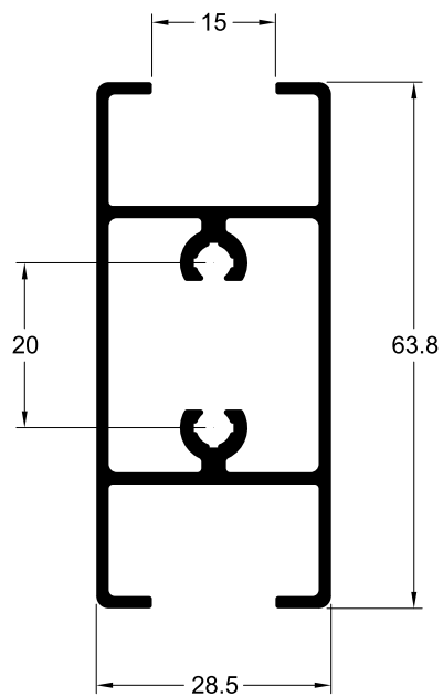
LG-34SB 0,957 Kg/m
