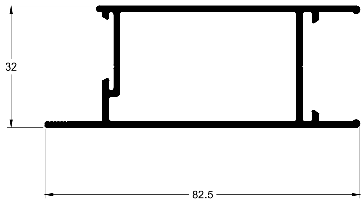
TLG-050A 0.925 Kg/m
