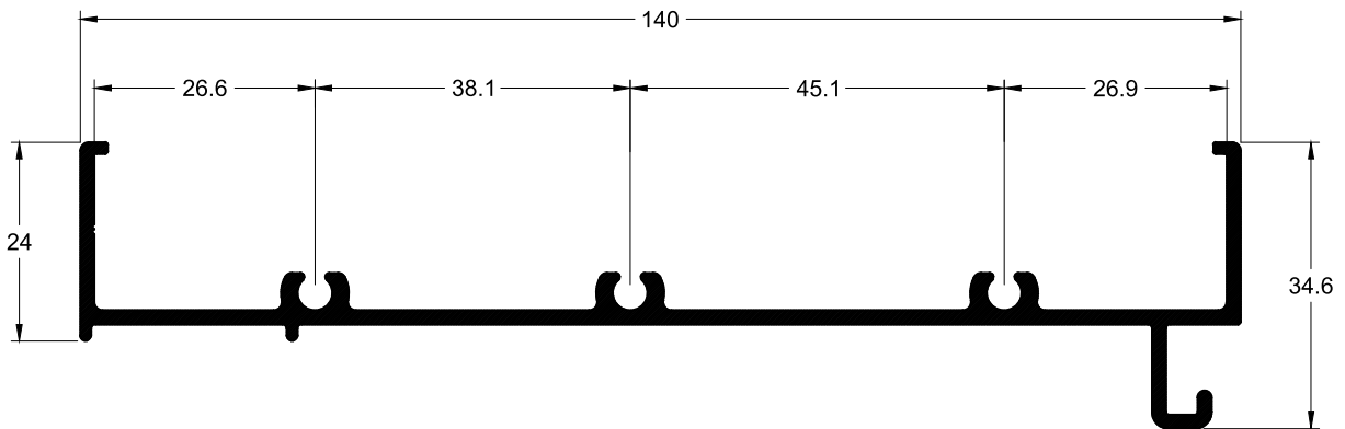
TLG-168A 1.117 Kg/m
