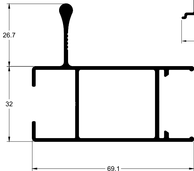
TLG-126A 0.959 Kg/m
