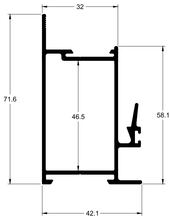
TLG-049A 0.978 Kg/m
