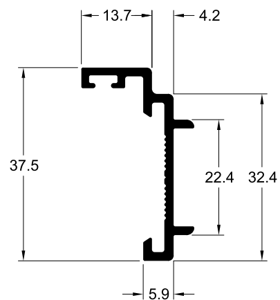
TLG-016 0.347 Kg/m
