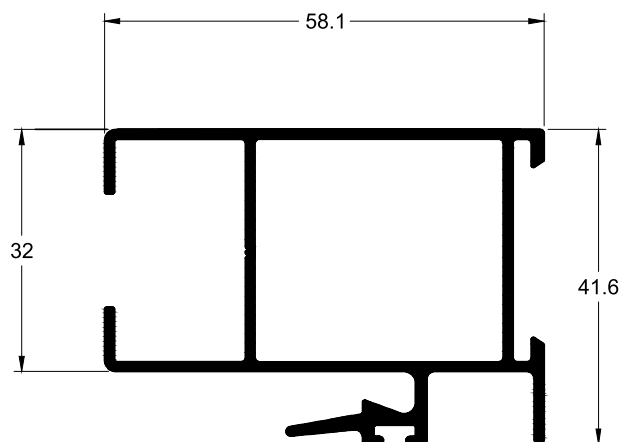
TLG-128 0.872 Kg/m
