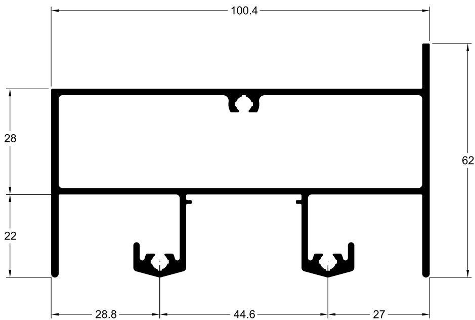
TLG-004 2.035 Kg/m
