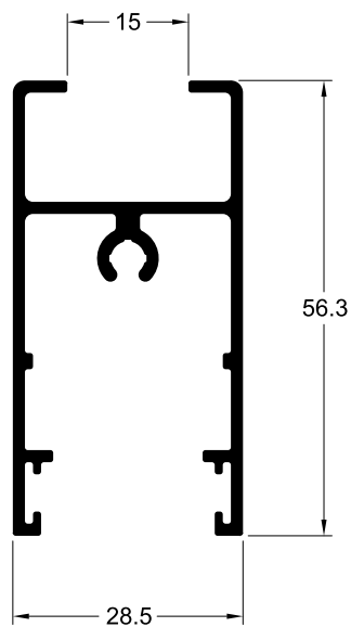
LG-06SB 0,759 Kg/m
