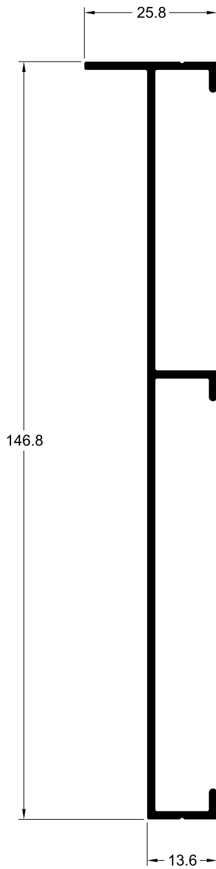
TLG-158 0.899 Kg/m
