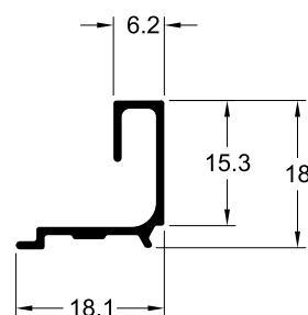
TLG-027 0.138 Kg/m
