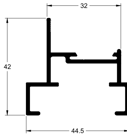
TLG-063 0.549 Kg/m
