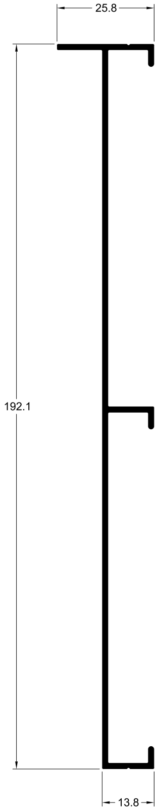
TLG-072 1.098 Kg/m
