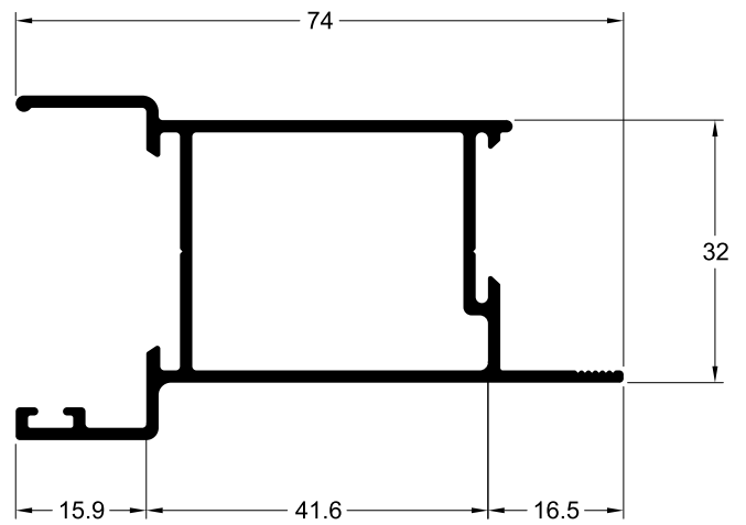
TLG-051 0.904 Kg/m
