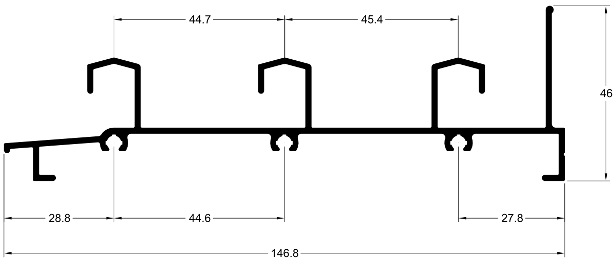
TLG-061 0.319 Kg/m
