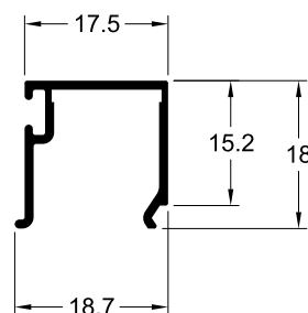
TLG-059 0.169 Kg/m
