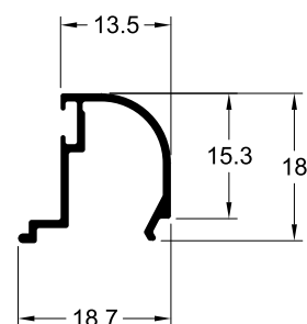
TLG-026 0.148 Kg/m
