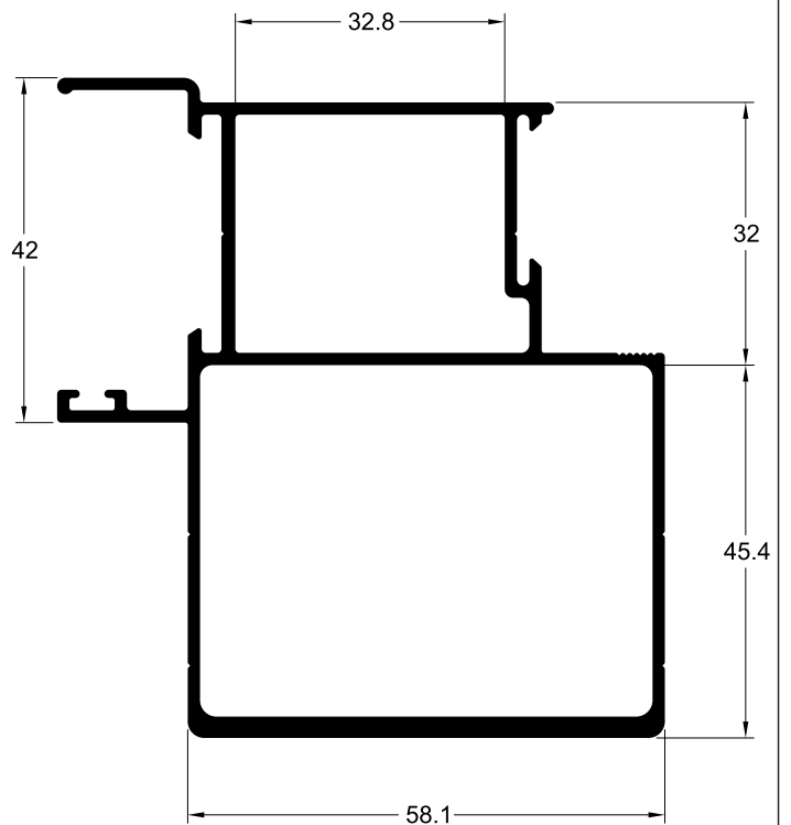
TLG-053 1.651 Kg/m
