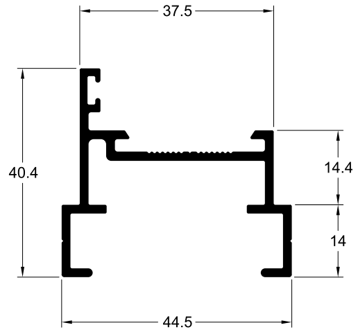
TLG-056C 0.642 Kg/m
