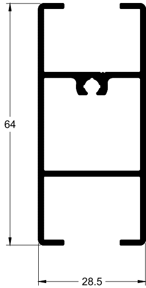
TLG-131A 0.764 Kg/m
