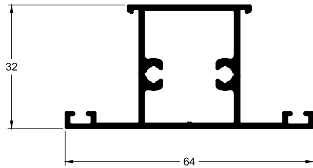
TLG-074 0.751 Kg/m
