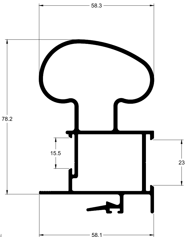
TLG-021 1.663 Kg/m
