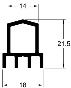
TLG-061 0.319 Kg/m
