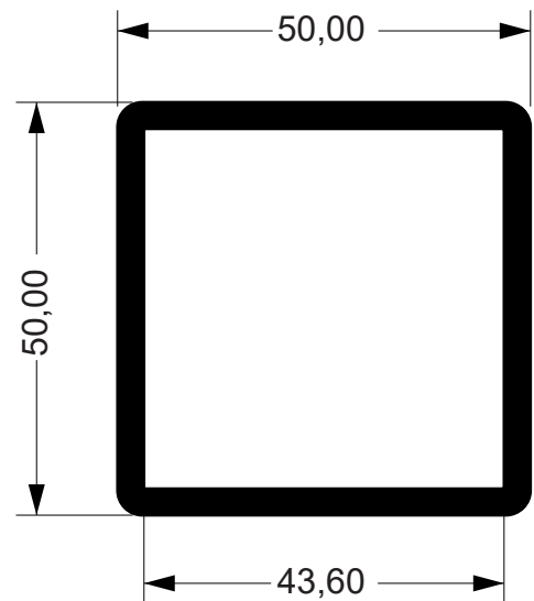
TQ-2006 3,188 kg/m
