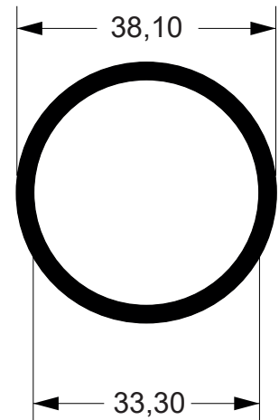
TR-0072 0,727 kg/m
