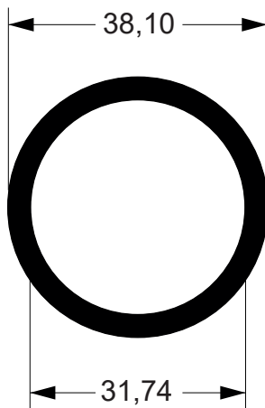
TR-0073 0,945 kg/m
