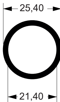
TR-0041 0,398 kg/m
